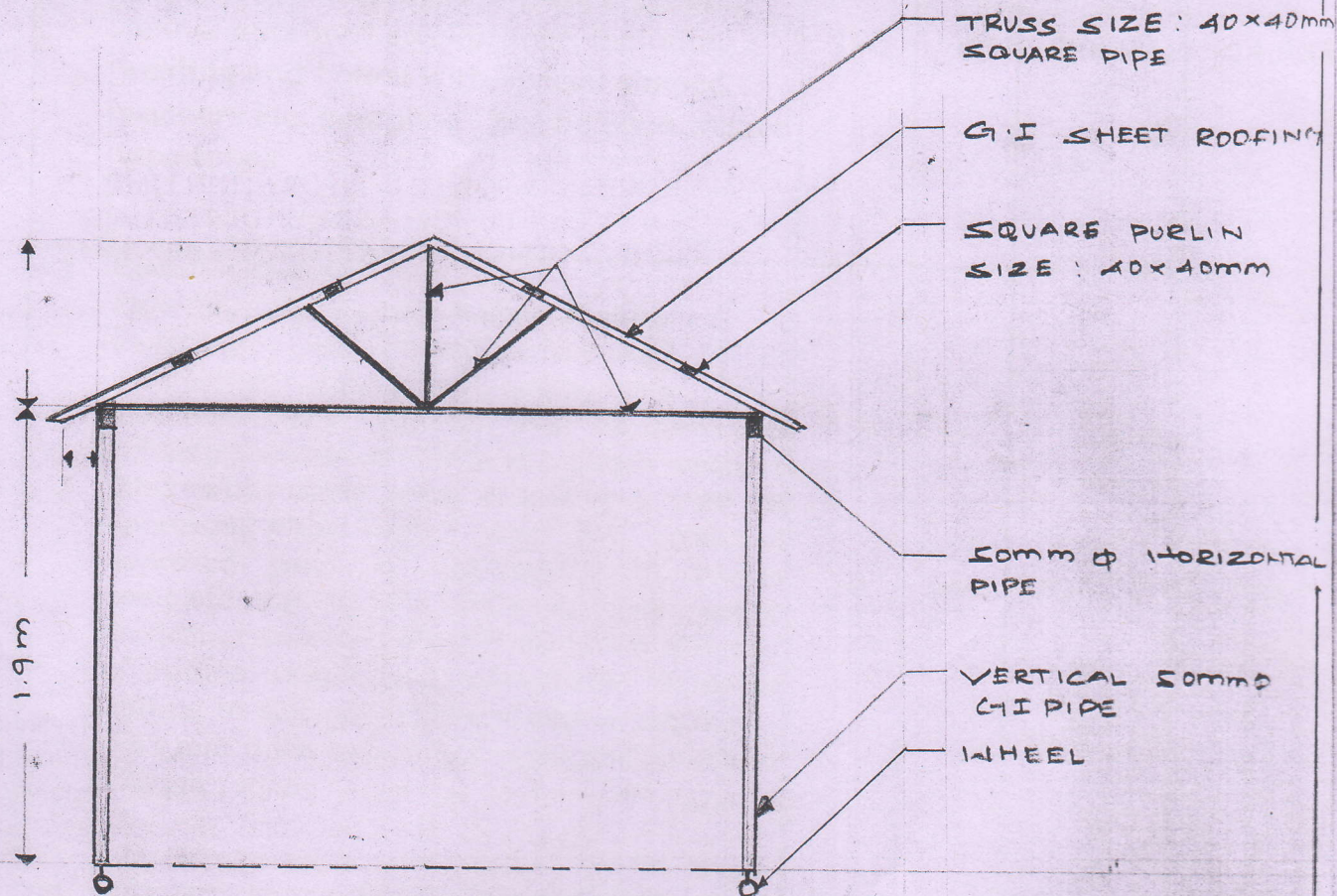
ELEVATION
